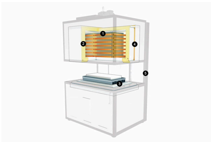
HB 钟罩炉内部结构
