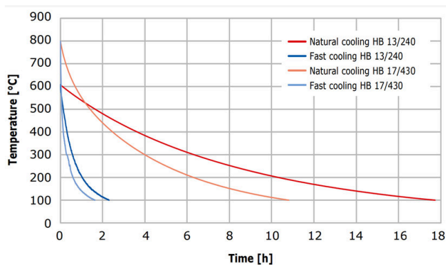
自然冷却と強制冷却のオプションの比較
