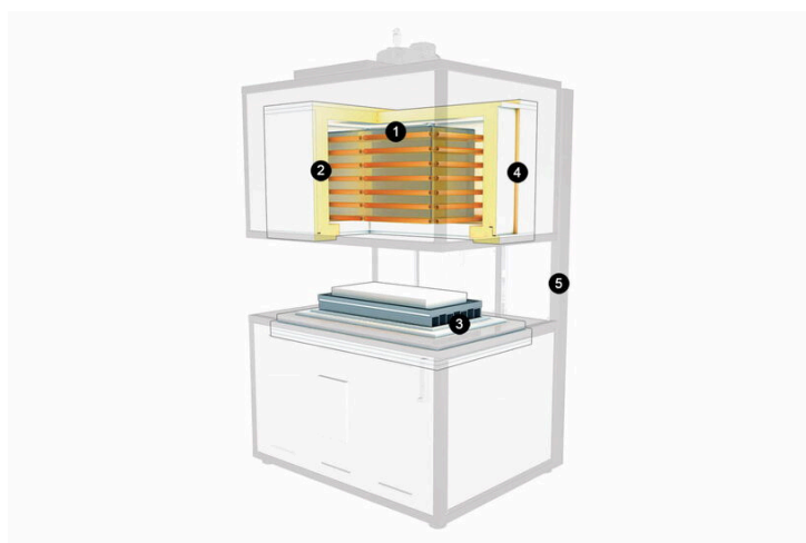
HBトップハット炉の内部を見る
