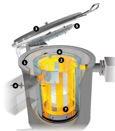
Vista interior LHTG
