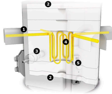
Vue de l'intérieur the HTRV-A split tube furnace
